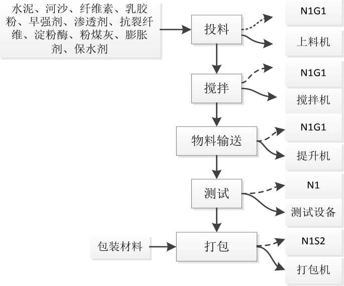
干粉砂浆主要生产工艺及产污节点
