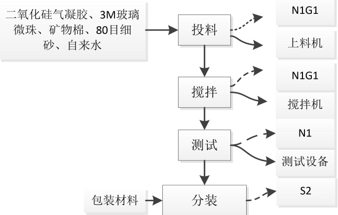
隔音砂浆主要生产工艺及产污节点
